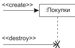
Рис. 9.28. Создание и уничтожение обобщенного объекта
