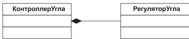
Рис. 8.13. Отношение агрегации по величине (композиция)
