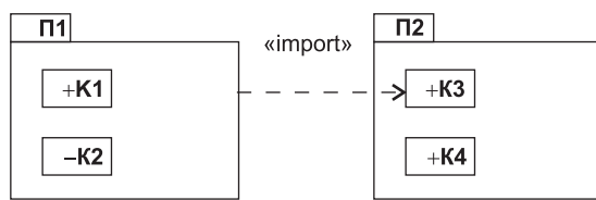
Рис. 10.8. Публичный импорт на уровне элемента пакета
