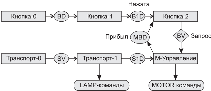
Рис. 7.8. Полная диаграмма системной спецификации
