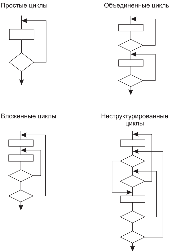
Рис. 14.15. Типовые структуры циклов
