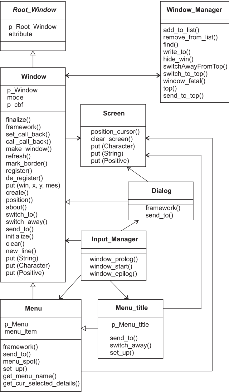
Рис. 13.19. Конечная диаграмма классов WUI
