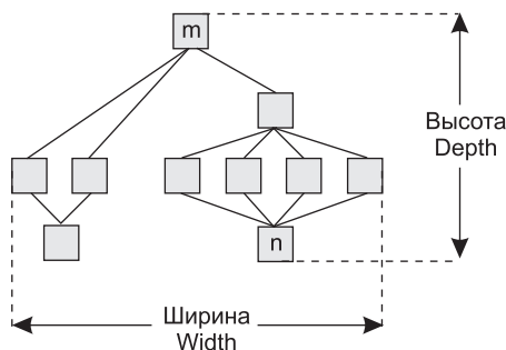
Рис. 6.21. Иерархическая структура программной системы
