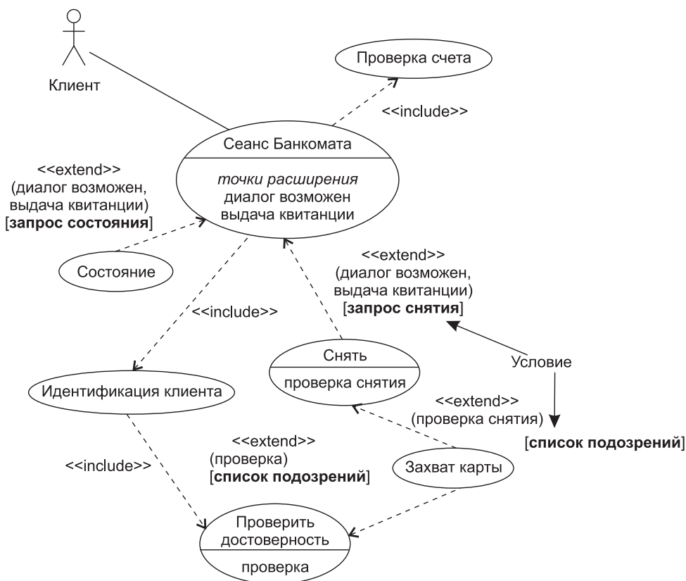
Рис. 9.10. Диаграмма Use Case для банкомата (с использованием включения и расширения)
