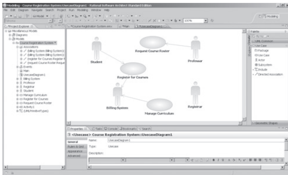
Рис. 19.20. Отношения между актерами и элементами Use Case
