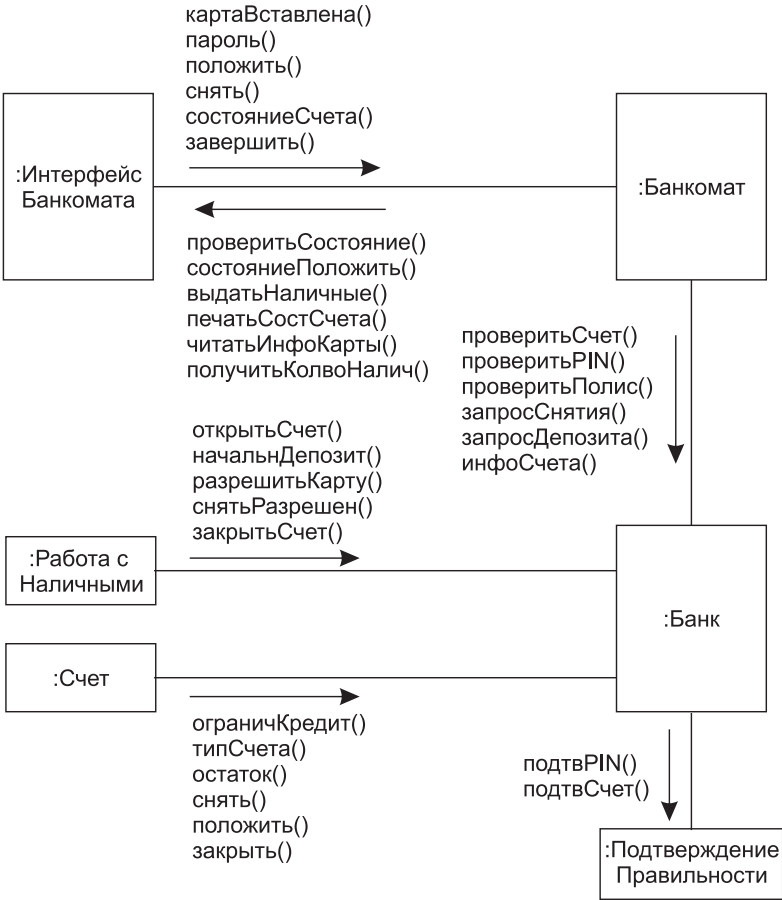
Рис. 17.1. Диаграмма коммуникации объектов банковской системы
