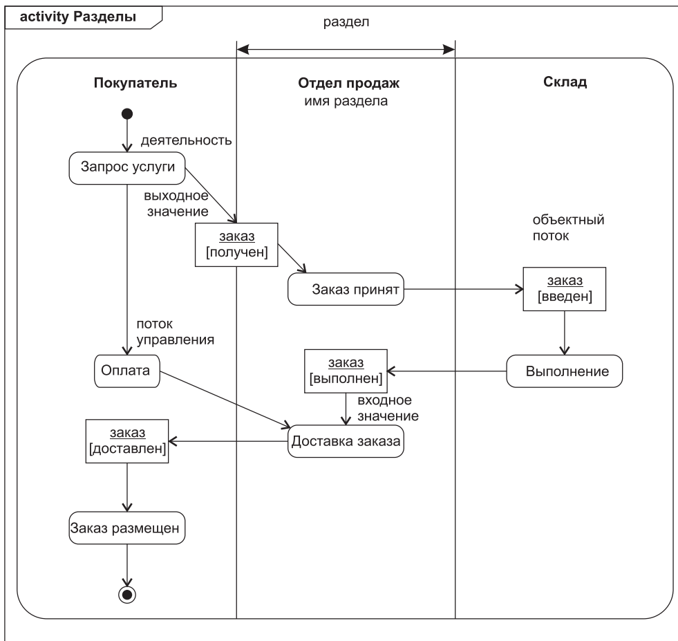
Рис. 9.20. Диаграмма деятельности с «плавательными дорожками»
