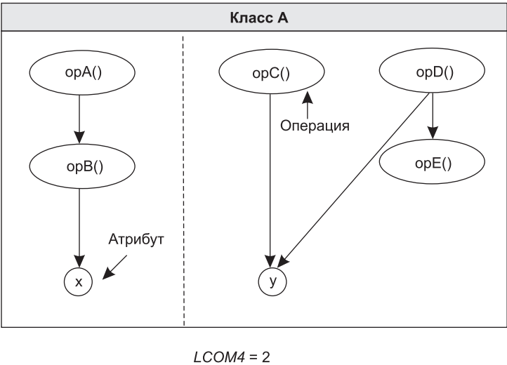
Рис. 12.5. Класс с плохой связностью
