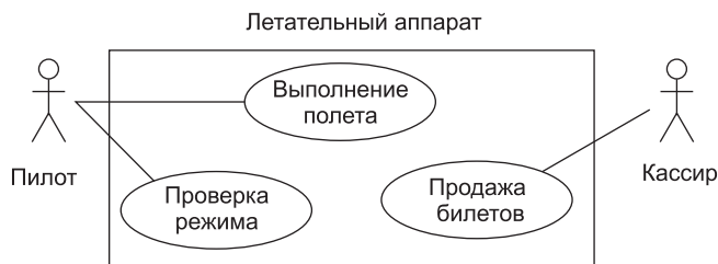
Рис. 9.2. Модель Use Case
