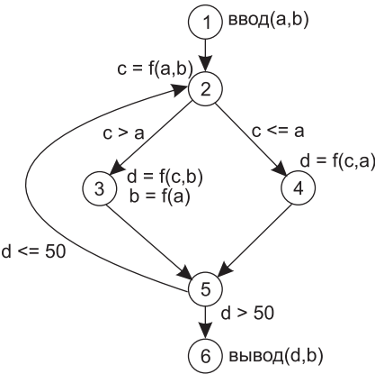
Рис. 14.12. Управляющий граф пятого объекта тестирования
