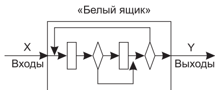
Рис. 14.3. Тестирование «белого ящика»
