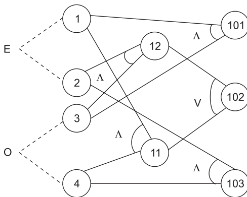
Рис. 15.14. Граф причинно-следственных связей
