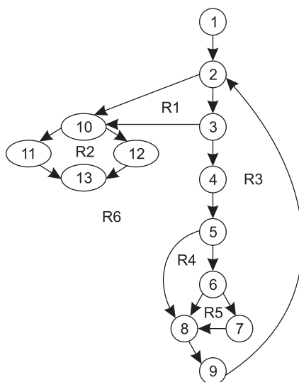
Рис. 14.7. Потокосный граф процедуры вычисления среднего значения
