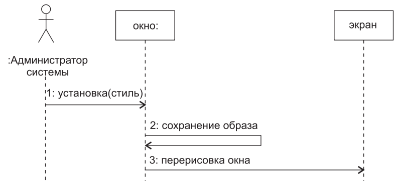
Рис. 13.11. Диаграмма последовательности Изменение стиля рамки
