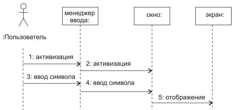
Рис. 13.13. Диаграмма последовательности Использование простого окна
