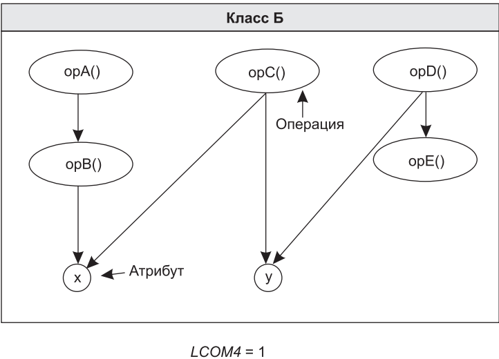
Рис. 12.6. Класс с хорошей связностью
