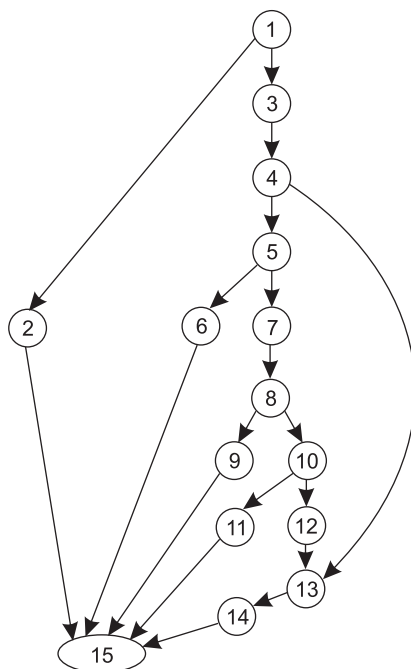
Рис. 14.9. Потокный граф второго объекта тестирования
