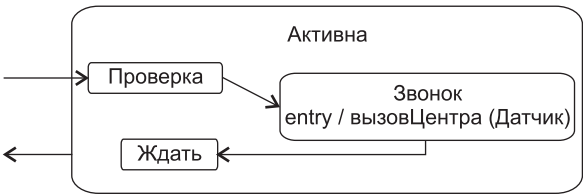
Рис. 9.42. Переходы в состоянии Активна
