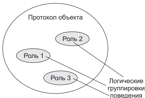
Рис. 8.3. Пространство поведения объекта
