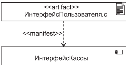
Рис. 10.68. Пример артефакта и реализуемого им компонента
