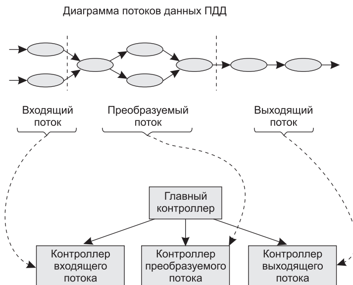
Рис. 7.3. Начальная структура ПС для потока «преобразование»
