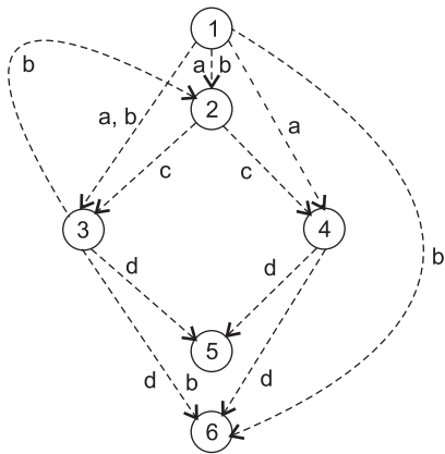
Рис. 14.13. Информационный граф пятого объекта тестирования
