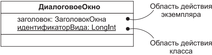
Рис. 10.17. Атрибуты уровней класса и экземпляра
