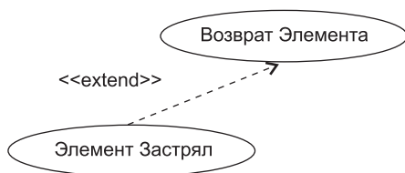
Рис. 9.13. Расширение элемента Use Case Возврат Элемента
