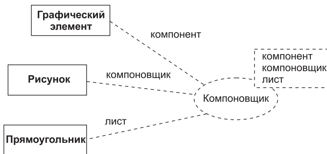
Рис. 10.49. Настройка паттерна Компоновщик
