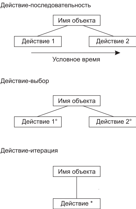
Рис. 5.13. Три типа структурных диаграмм Джексона
