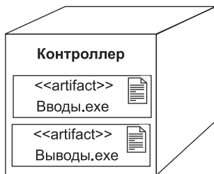
Рис. 10.71. Размещение артефактов внутри узла
