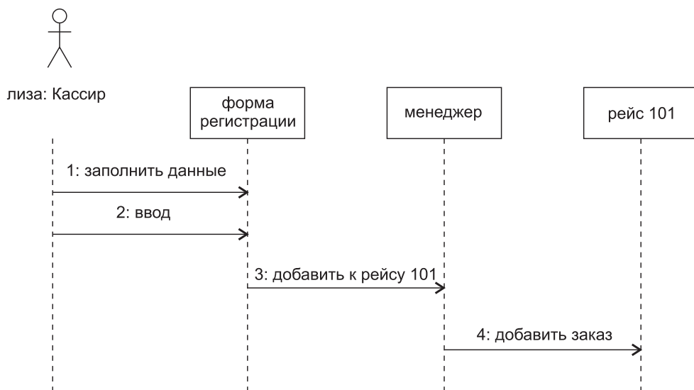
Рис. 10.39. Динамическая составляющая кооперации Заказ авиабилета
