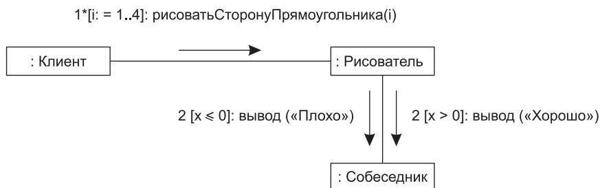
Рис. 9.25. Итерация и ветвление
