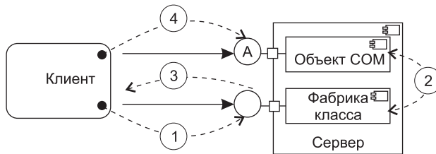
Рис. 10.63. Создание COM-объекта с помощью фабрики класса. Клиент вызывает IClassFactory::createInstance (IID A) (1); фабрика класса создает COM-объект и получает указатель на его интерфейс (2); фабрика класса возвращает указатель на интерфейс A COM-объекта (3); теперь клиент может вызывать операции COM-объекта (4)
