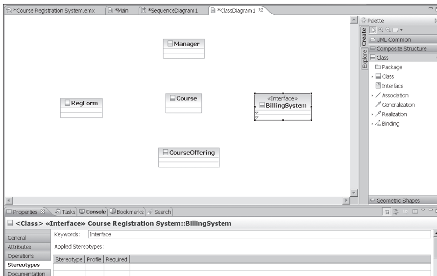
Рис. 19.35. Класс Billing System после введения стереотипа Interface
