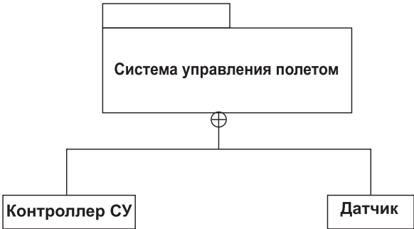
Рис. 10.3. Внешнее обозначение содержимого пакета
