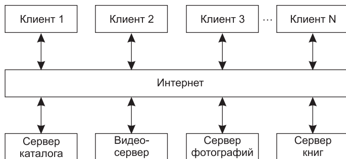
Рис. 6.6. Клиент-серверная архитектура сетевой библиотеки
