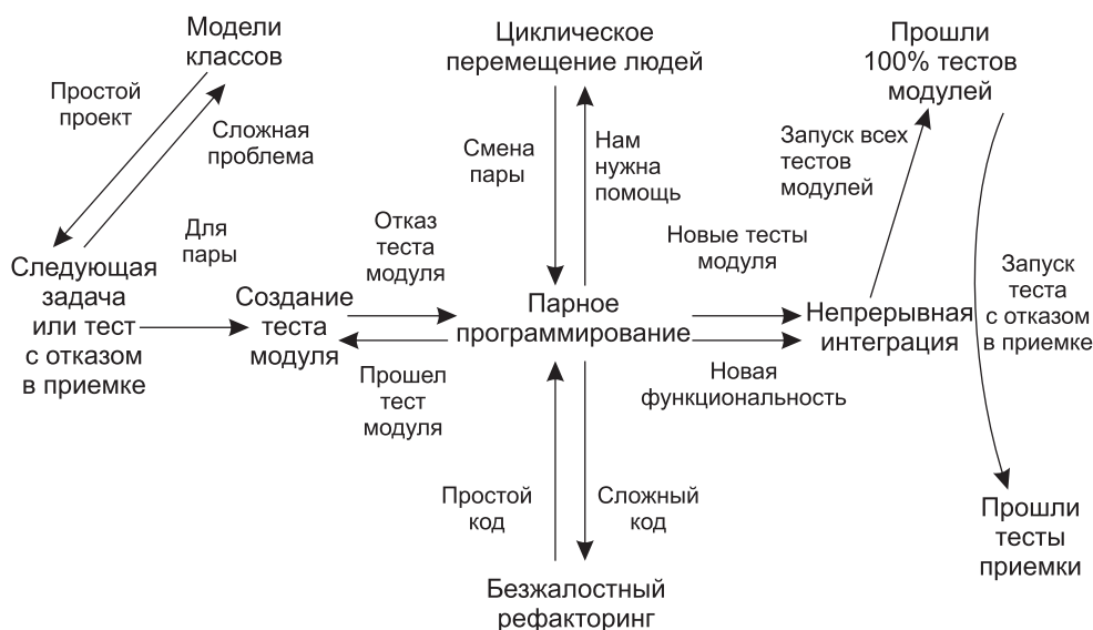
Рис. 13.34. Организация коллективного владения кодом
