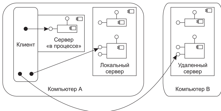
Рис. 10.61. Различные серверы СОМ-объектов
