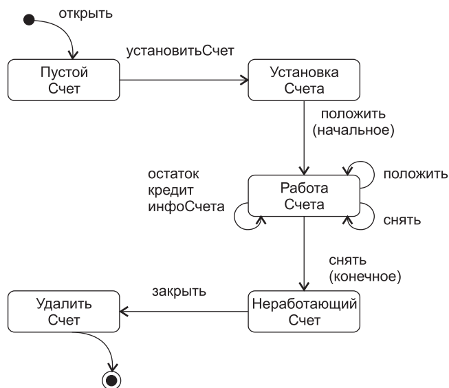
Рис. 17.2. Диаграмма конечного автомата класса Счет
