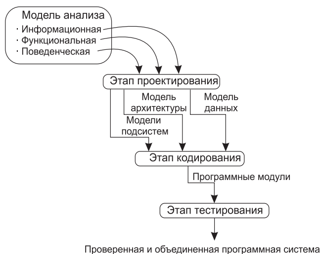
Рис. 6.1. Информационные потоки процесса синтеза ПС
