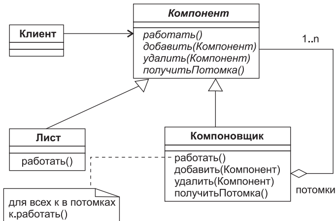
Рис. 10.47. Структурная составляющая паттерна Компоновщик
