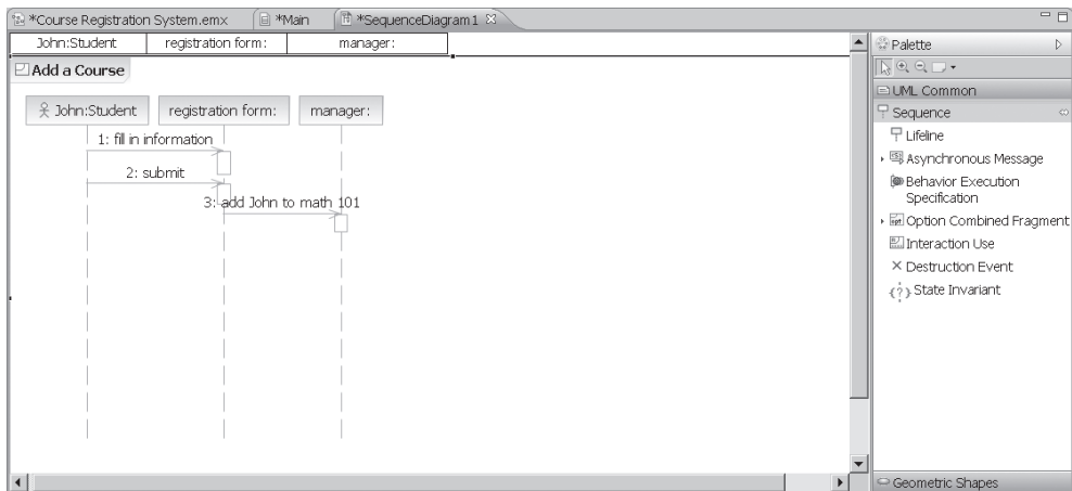
Рис. 19.26. Диаграмма последовательности после добавления manager
