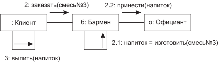
Рис. 9.23. Поток синхронных сообщений
