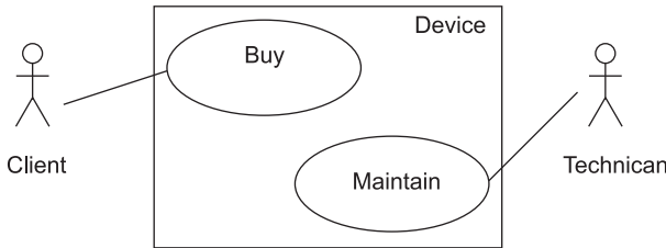
Рис. 13.20. Начальная диаграмма Use Case
