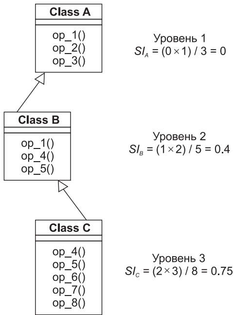
Рис. 12.8. Расчет индексов специализации классов
