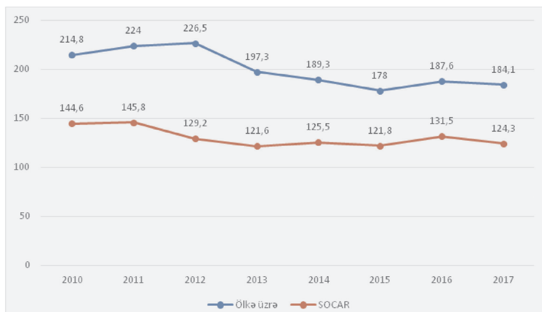
Diaqram 1. Çirkləndirici maddələrin ölkə və SOCAR üzrə dəyişmə dinamikası (2010-2017 il), min ton
