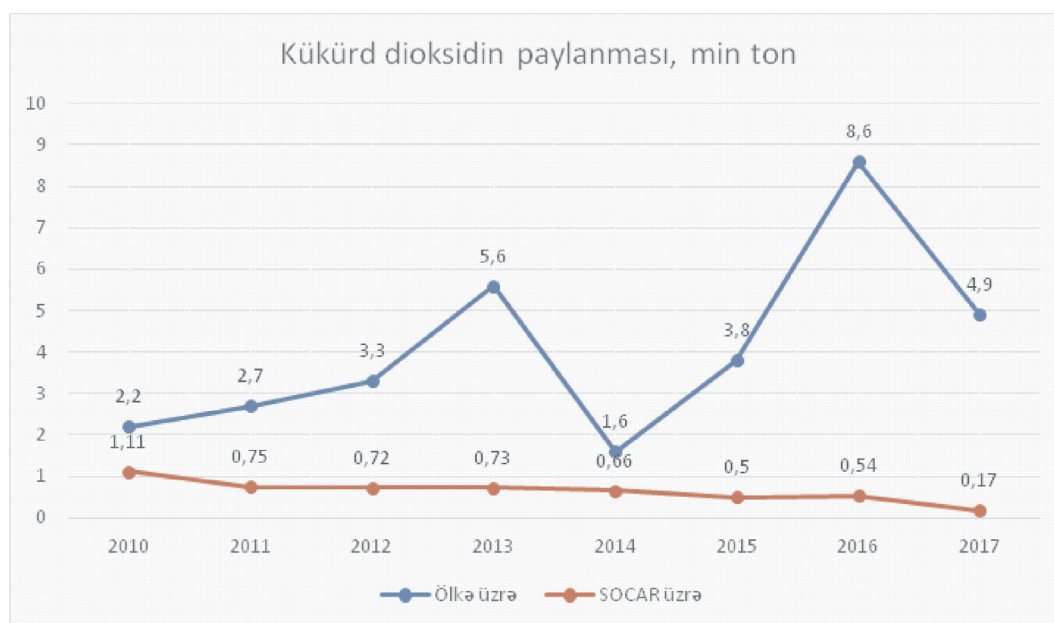
Diaqram 3. Kükürd dioksidin dəyişmə dinamikası, min ton
