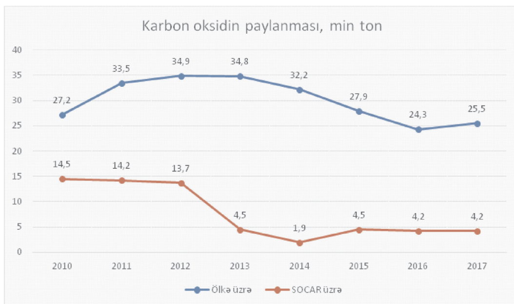
Diagram 5. Karbon oksidin dəyişmə dinamikası, min ton
